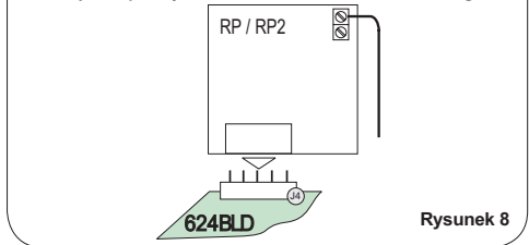
Przykład podłączenia modułu sterowania radiowego
